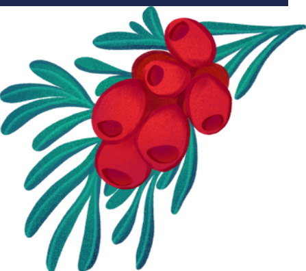
Yew
